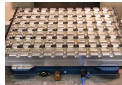
*VM300 真空吸盤 (45175) 和 VM300 (45130)
