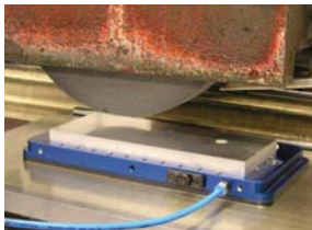
*真空吸盤VM100 (45375) 在磁盤上
